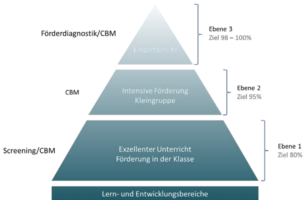
Abbildung 10: Mehrebenenpräventionskonzept 19
